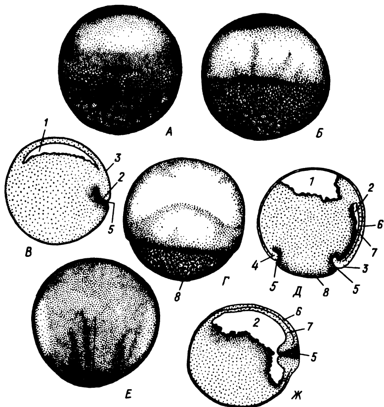
Рис. VII.3. III этап — гастрюляция у осетра (по Гинзбург, Детлаф, 1975). А — появление темной полоски, Б — ранняя гастрюла. В — то же в разрезе, Г — поздняя гастрюла, Д — то же в разрезе, Е — замыкание бластопора, Ж — то же в разрезе. 1 — бластоцель, 2 — гастрюцель, 3 — верхняя губа бластопора, 4 — нижняя губа бластопора, 5 — бластопор, 6 — наружный слой, 7 — внутренний слой, 8 — желточная пробка
