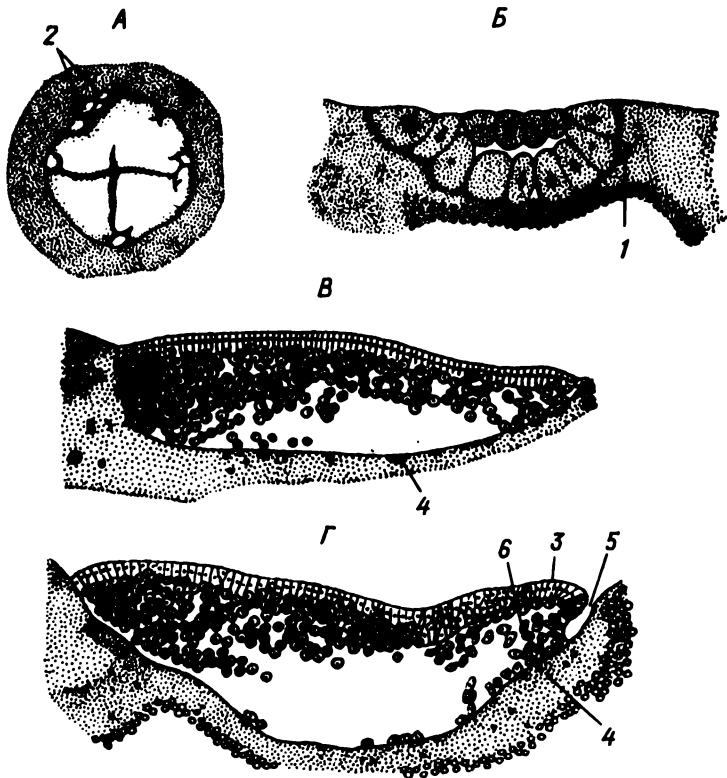
Рис. IX.1. Ранние стадии развития ската Torpedo (по Рюккерт из Иванова, 1945). А — стадия 4 бластомеров; Б — стадия 64 бластомеров на разрезе; В — эпителиальная бластула; Г — начало гастрюляции (передний край слева). 1 — ядра избыточных спермиев, 2 — ложные бластомеры, 3 — верхняя губа бластопора, 4 — перибласт, 5 — гастрюцель, 6 — энтодерма
