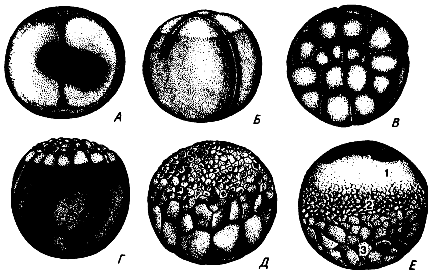
Рис. VII.2. II этап — дробление яйца осетра (по Гинзбург, Детлаф, 1975). А — первое деление (вид сверху), Б — второе деление, приводящее к образованию 4 бластомеров, В — четвертое деление (вид сверху), Г — седьмое деление, Д — ранняя бластула, Е — поздняя бластула. 1 — микромеры, 2 — краевая зона, 3 — макромеры
