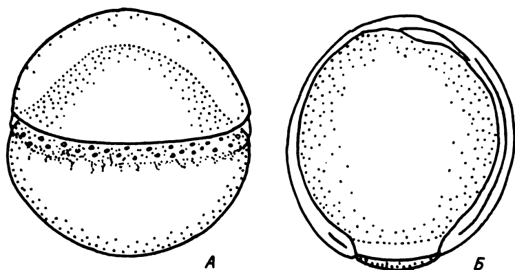
Рис. VIII.3. IV этап — гастрюляция у карпа (ориг.). А — начало обрастания (7 ч), Б — завершение обрастания, заметны закладка тела зародыша и небольшая желточная пробка (9 ч)
