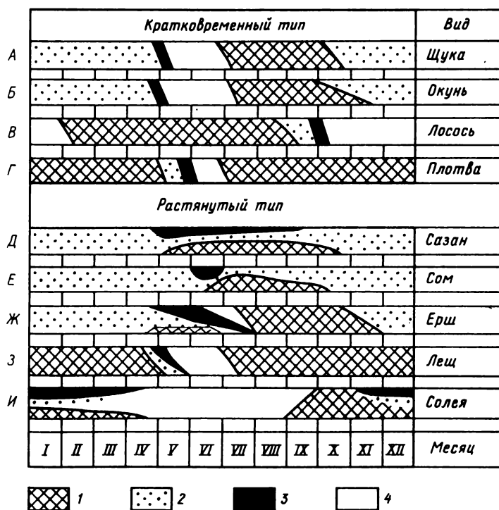
Рис. IV.2. Половые циклы самцов с различными типами вымета спермы (по Буцкой, 1975; соля — по Заки, 1989). 1 — волна сперматогенеза, 2 — спермии в семенных каналцах, 3 — вымет спермиев, 4 — посленерестовое состояние семенников
