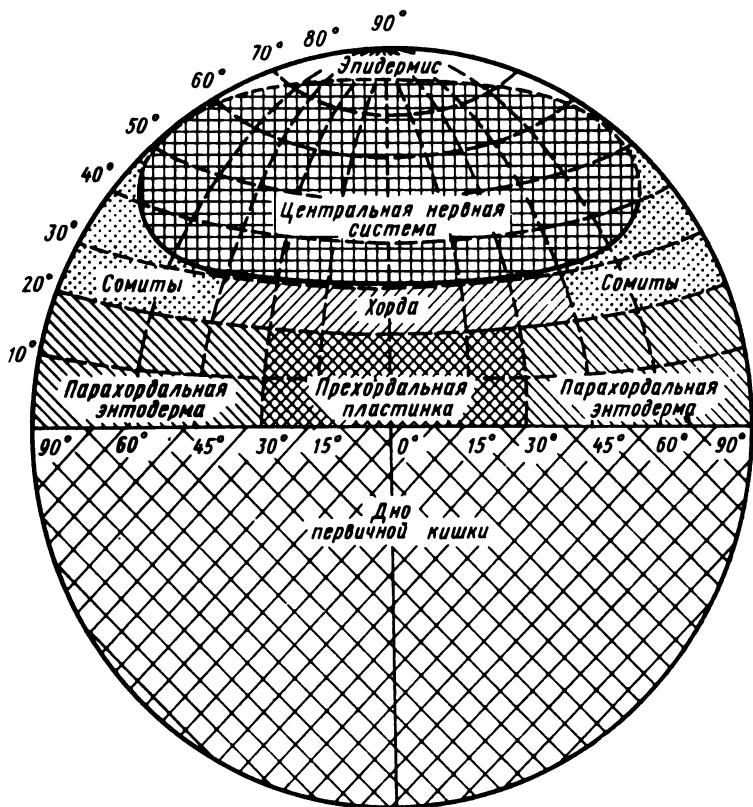
Рис. VII.4. Карта расположения презумптивных зачатков на стадии поздней бластулы у осетра и севрюги (по Ballard, Ginsburg, 1980 из Детлаф и др., 1981)
