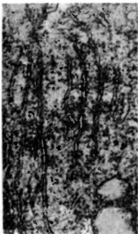
Рис. II.5. Пористые пластинки в цитоплазме ооцит белого толстолобика (фото Емельяновой)
