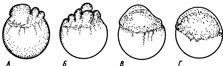
Рис. V.2. Изменения неоплодотворенных яиц белого толстолобика (ориг). А, Б — ложное дробление; В—Г — ложное обрастание
