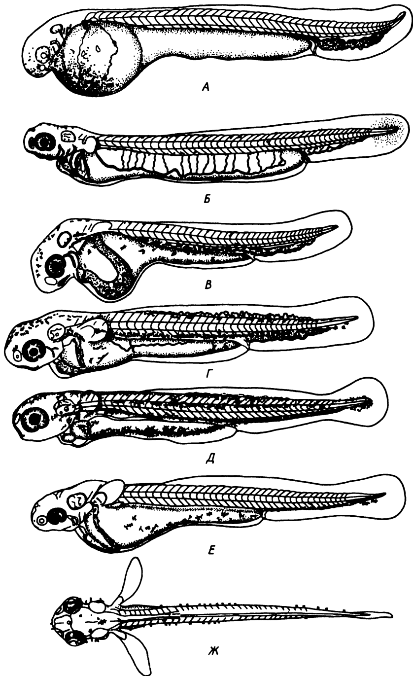
Рис. X.1. Зародыши и предличинки карповых рыб разных экологических групп (по Крыжановскому, 1949). Литофильная группа: А, Б — гокчинский усач; Фитофильная группа: В, Г — сазан, Д — верховка; псаммофильная группа: Е, Ж — пескарь
