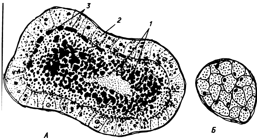
Рис.11.9. Резорбция желтковых ооцитов (ориг.) А — начало резорбции; Б — атретическое тело. 1 — желток, 2 — фолликулярные клетки с включениями, 3 — фрагменты лучистой оболочки
