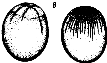
Рис. VII.13. Яйцевая оболочка (А) и дробление яиц ильной рыбы (Б) и панцирника (В). 1 — лучистая оболочка, 2 — нити хориона, 3 — они же, сильно растянувшиеся после прилипания к растению (4). (А — из Nelsen, 1953; Б, В — из Гинзбург, 1968)
