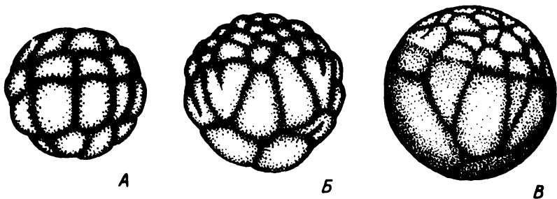
Рис. VII. 11. Дробление яиц рогозуба (А), протоптеруса (Б) и чешуйчатника (В) (А, Б — из Гинзбург, 1968; В — по Kerr, 1901)
