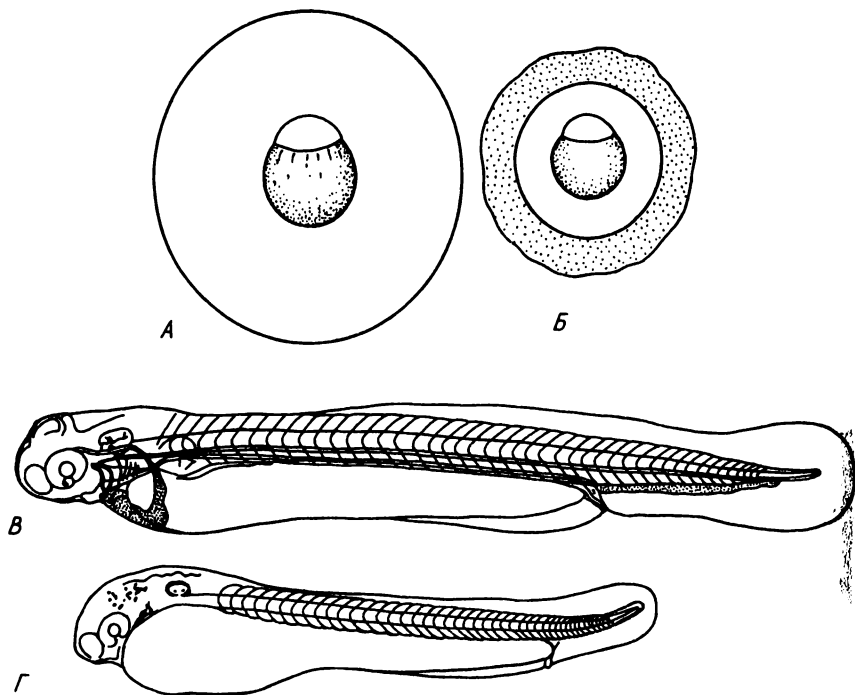
Рис. X.2. Икра и предличинки пресноводных пелагофильных рыб. А — белого толстолобика, Б — чебаковидного пескаря (по Соину, 1968), В — черного амура (по Сухановой, 1967), Г — востробрюшки (по Крыжановскому, 1949)
