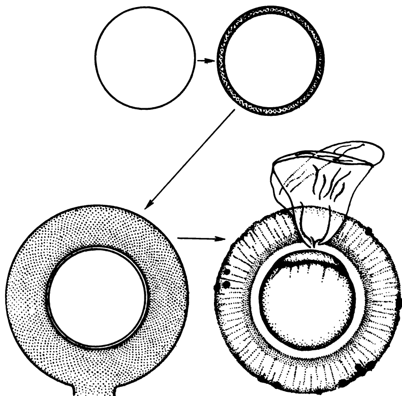
Рис. II.17. Образование клейкой оболочки икринки лжепескаря Pseudogobio rigularis (ориг.). Происходит сползание тонкой лучистой оболочки с плотного слизистого содержимого перивителлинового пространства, которое становится липкой перивителлиновой оболочкой.
