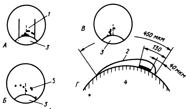
Рис. I. 1. Расположение первичных половых клеток (5) у зародышей медаки на стадии гастролы (по Gamo, 1961). А—В — вид со спины, Г — вид сбоку. 1 — область закладки зародыша, 2 — зародыш, 3 — желточная пробка, 4 — желточный мешок
