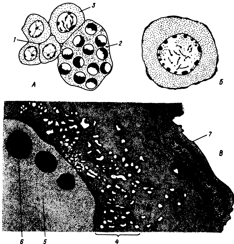
Рис. 11.2. Оогонии и ооциты периода превителлогенеза у белого толстолобика (ориг.). А — оогонии (1), ооциты стадии зиготены (2) и пахитены (3); Б — ооцит стадии ранней диплотены; В — размножение митохондрий (4) в околоядерной зоне, 5 — ядро, 6 — ядрышки, 7 — фолликулярная клетка
