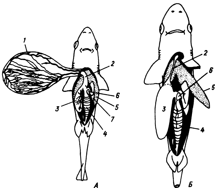
Рис. IX.4. Перемещение желтка из наружного желточного мешка во внутренний у зародышей колючей акулы (по Te Winkel, 1943). А — длина 170 мм, Б — длина 230 мм. 1 — наружный желточный мешок с желточными сосудами, 2 — желточный канатик, 3 — внутренний желточный мешок, 4 — спиральная кишка, 5 — печень, 6 — поджелудочная железа, 7 — селезенка
