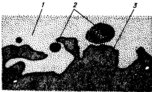
рис. 11.4. Извилистость мембраны ядра ооцита белого толстолобика (рис. по фото Емельяновой). 1 — фрагмент ядра, 2 — ядрышко, 3 — цитоплазма
