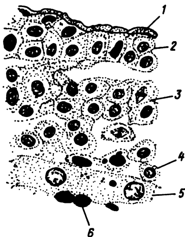
Рис. VIII.5. Срез через зародышевый щиток карпа (ориг.). 1 — перидерма, 2 — эктодерма, 3 — мезодерма, 4 — энтодерма, 5 — перибласт, 6 — желток
