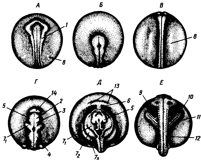
Рис. VII.5. IV этап — развитие зародыша осетра от конца гастрляции до начала пульсации сердца (по Гинзбург, Детлаф, 1975). А — стадия широкой нервной пластинки; Б, В — стадия поздней нейрулы — смыкание нервных валиков и образование нервной трубки (Б — головной, В — спинной отделы); Г — образование трех мозговых пузырей; Д — слияние боковых пластинок и закладка сердца; Е — развитие предпочки. 1 — нервные валики; 2 — передний, 3 — средний, 4 — задний мозговые пузыри; 5 — зачатки глаз, 6 — сердце, 7 — зачатки жаберных дуг (7 1 — первой, 7 2 — второй, 7 3 — третьей пары); 8 — зачаток выделительной системы, 9 — почечные канальцы, 10 — собирательный канал, 11 — выносящий канал, 12 — сомиты, 13 — боковая пластинка, 14 — железа вылупления
