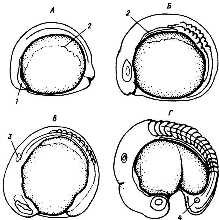
Рис. VIII.7. V этап — органогенез у карпа (ориг.). А — закладка зародыша (около 10 ч), Б — появление зачатков глаз (13 ч), В — появление слуховых плакод (15 ч), Г — появление в глазах хрусталиков, полостей в слуховых зачатках и купферова пузырька (18—20 ч). 1 — головная мезодерма, 2 — боковая пластинка, 3 — слуховая плакода, 4 — купферов пузырек
