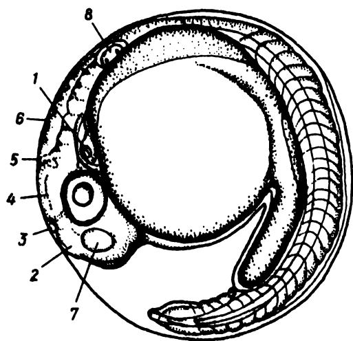
Рис. VIII.8. VI этап развития карпа — отчленение хвостового отдела от желточного мешка (1 сут 6—8 ч) (ориг.). 1 — сердце, 2 — передний мозг, 3 — эпифиз (область промежуточного мозга), 4 — средний мозг, 5 — зачаточный мозжечок, 6 — продолговатый мозг (заметны энцефаломеры), 7 — обонятельная капсула, 8 — слуховой пузырек (видны отолиты).
