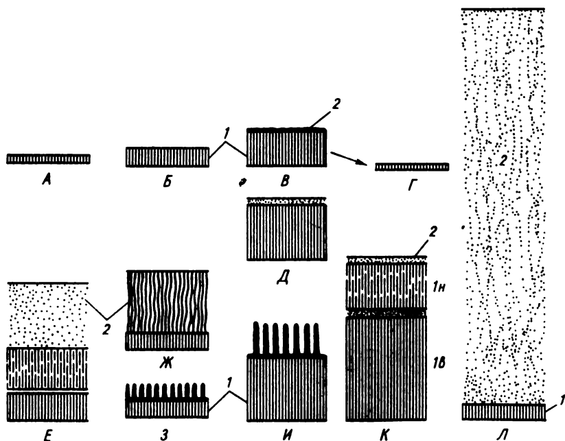
Рис. 11.14. Оболочки яиц рыб (ориг.). А — камбала-ершоватка, Б — треска (до набухания), В — белый толстолобик (до набухания), Г — то же (после набухания), Д — карп, Е — пинагор, Ж — большеротый буффало, З — обыкновенный пескарь, И — плотва, К — севрюга, Л — каналный сом. 1 — лучистая оболочка (1в — внутренняя, 1н — наружная), 2 — хорион
