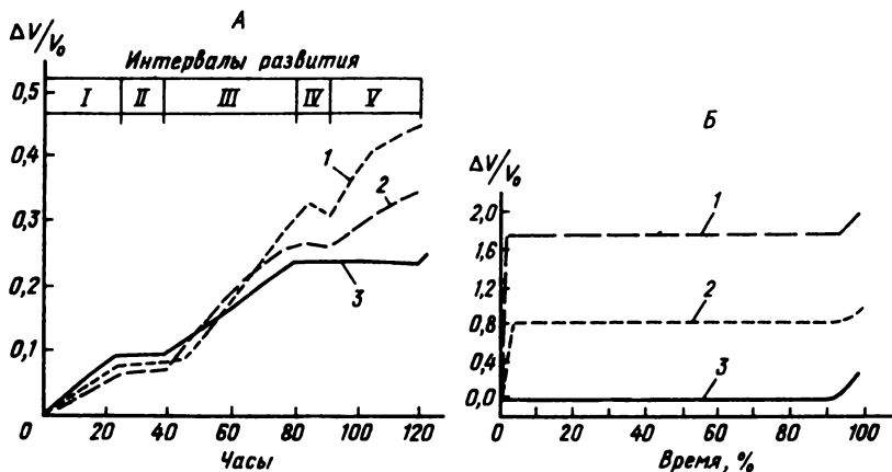
Рис. VI.1. Потребление воды из внешней среды развивающимися яйцами осетровых (А) и костистых (Б) рыб (по Зотину, 1961). \Delta V — объем поступившей или вышедшей из яйца воды, V_0 — начальный объем яйца. А — осетровые рыбы: 1 — осетр, 2 — белуга, 3 — севрюга.
