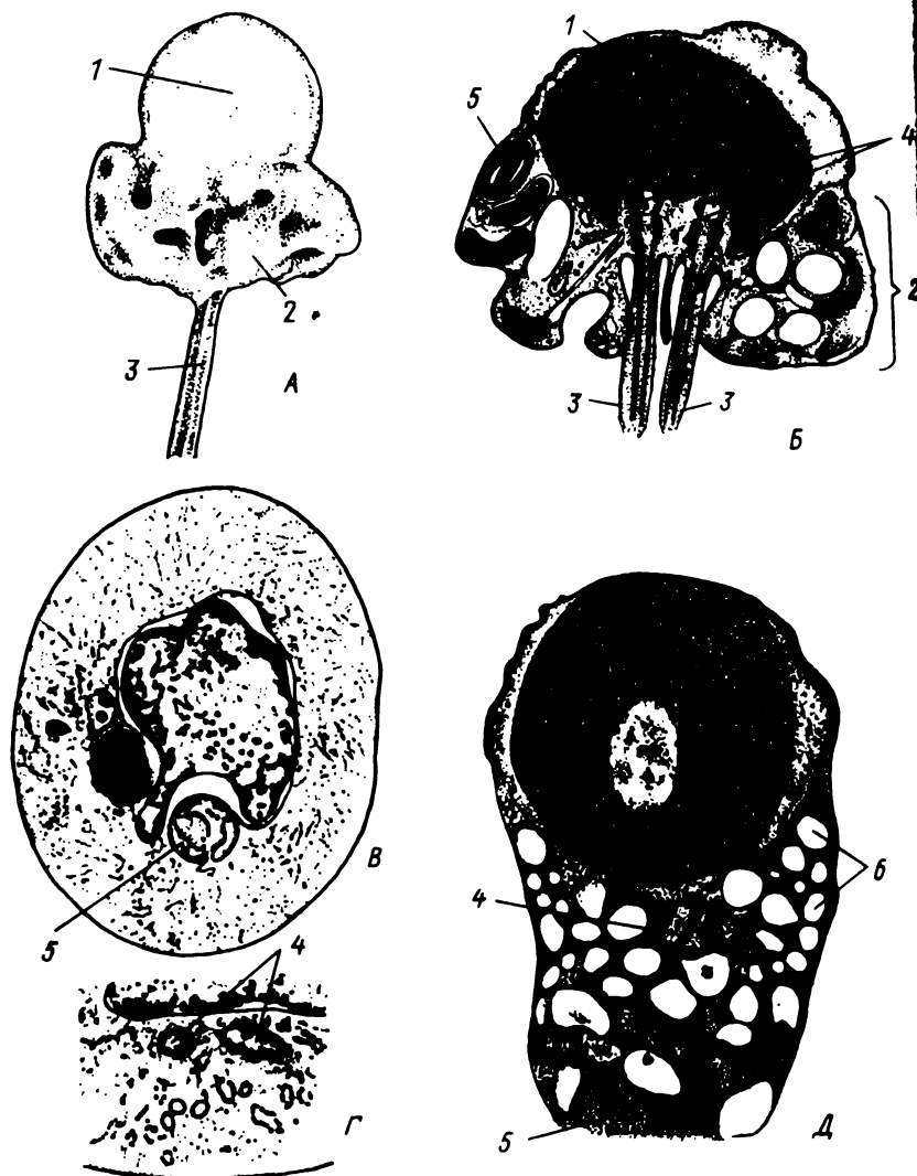
Рис. III.5. Необычные сперматозоиды костистых рыб: А, Б — канального сома (А — сканирующая, Б — просвечивающая электронная микроскопия) (по Емельяновой, Макеевой, 1991); В, Г — гимнарха (по Mattei et al., 1967); Д — петроцефалюса Petrocephalus (по Mattei et al., 1972). 1 — головка, 2 — средняя часть, 3 — жгутик, 4 — центриольный аппарат, 5 — митохондрия, 6 — пузырьки эндоплазматической сети
