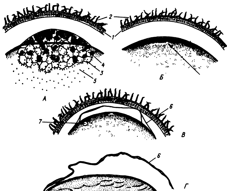
Рис. VIII.11. Ранние стадии развития нотобранха Nothobranchius guentheri (по Авни, Соину, 1974). А — начало обрастания и дисперсии глубоких клеток (возраст 30 ч), Б — начало агрегации клеток (отмечено стрелкой) (3,5 сут), В — образование тела зародыша (9,5 сут), Г — экстраэмбриональная мембрана. 1 — лучистая оболочка, 2 — хорион, 3 — перидерма, 4 — глубокие клетки, 5 — ядра перибласта, 6 — экстраэмбриональная мембрана, 7 — купферов пузырек
